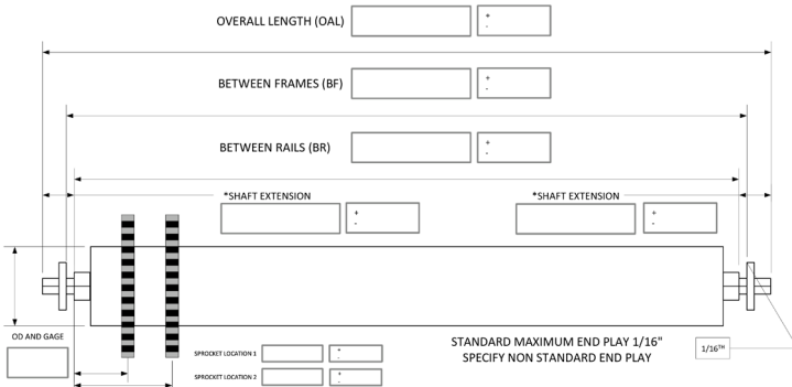
SPROCKET ROLLER
